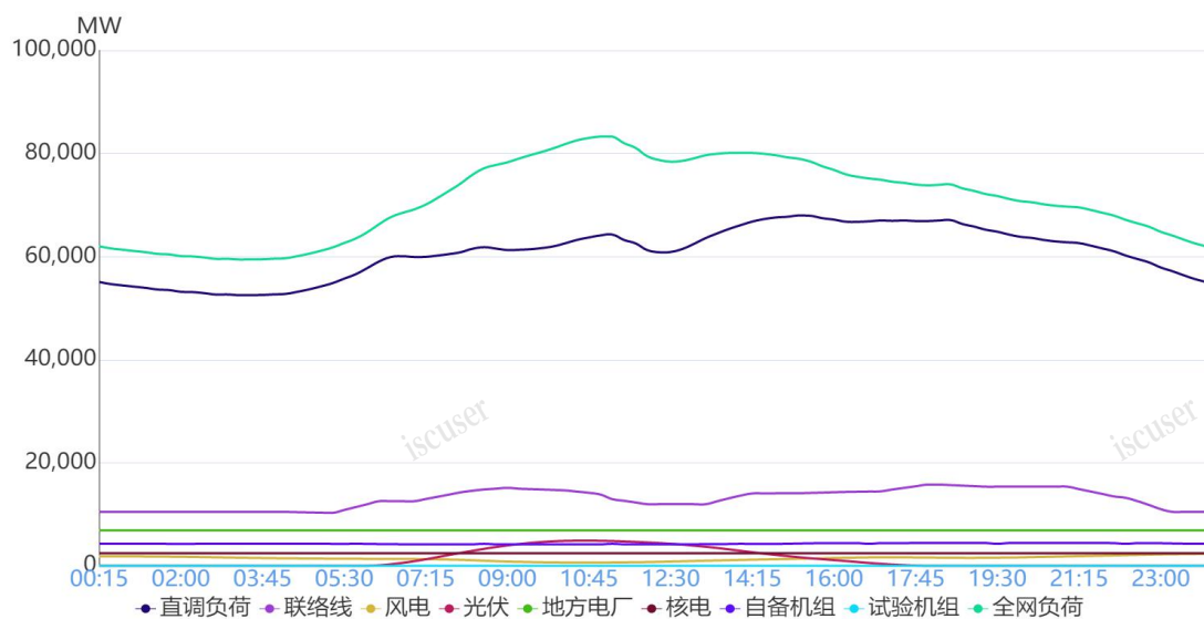
图 1 9月27日负荷及电源出力预测情况
