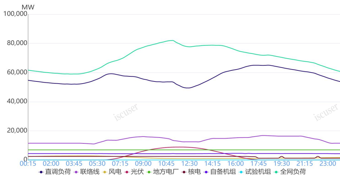
图 1 9月28日负荷及电源出力预测情况
