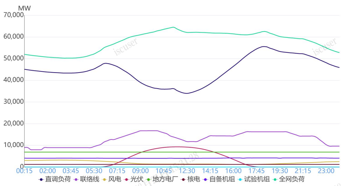
图1 10月1日负荷及电源出力预测情况
