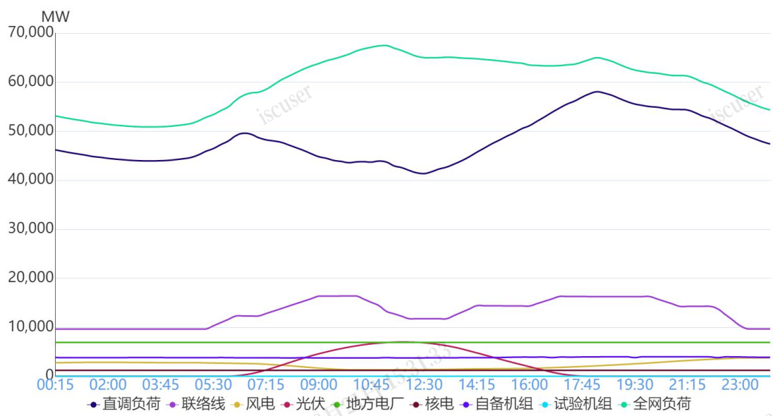
图 1 10月2日负荷及电源出力预测情况
