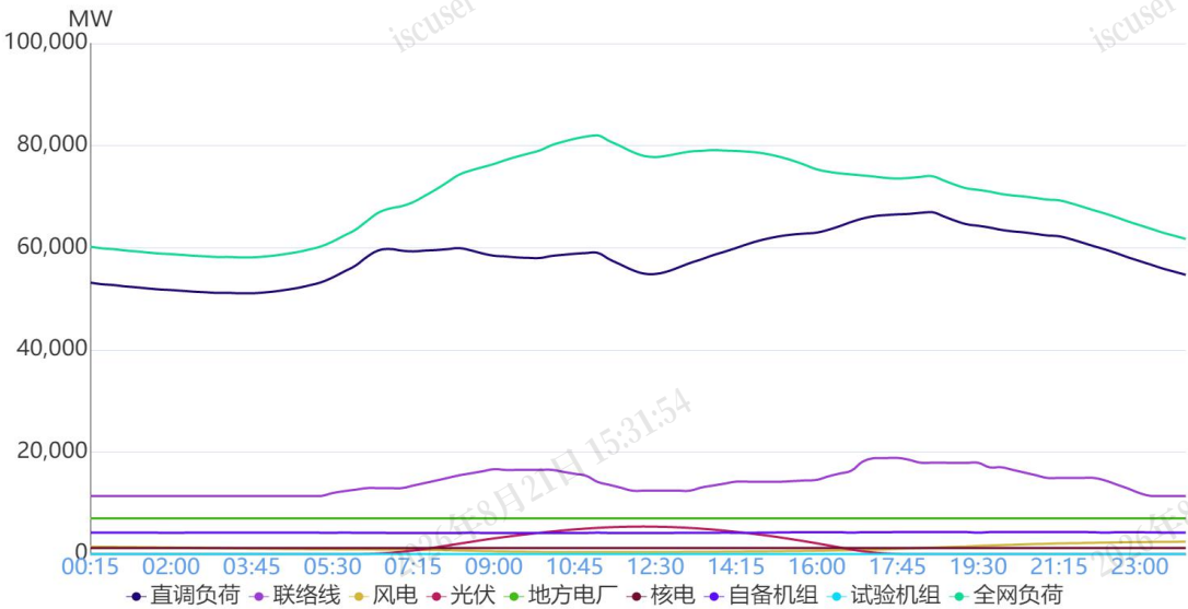
图1 10月7日负荷及电源出力预测情况
