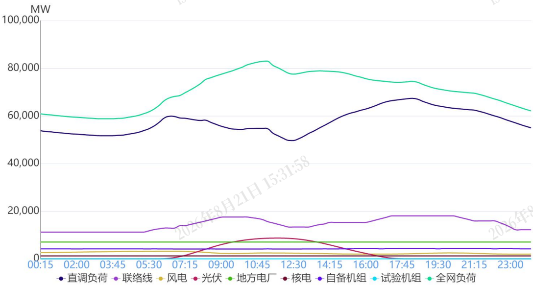
图1 10月8日负荷及电源出力预测情况
