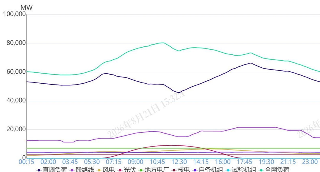
图1 10月9日负荷及电源出力预测情况
