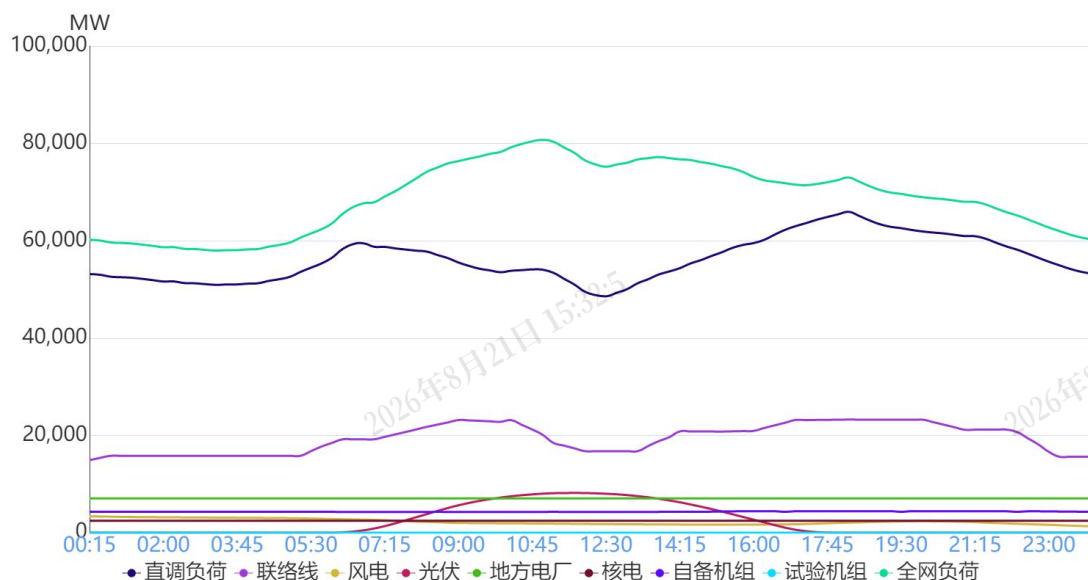
图1 10月10日负荷及电源出力预测情况
