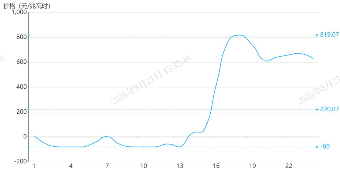
图 2 10 月 20 日日前市场用电侧价格
