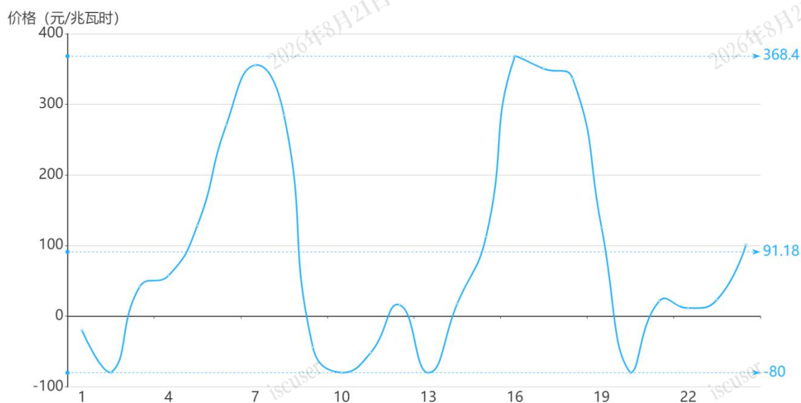
图3 10月23日实时市场用电侧价格
