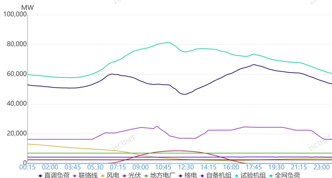
图 1 10月24日负荷及电源出力预测情况
