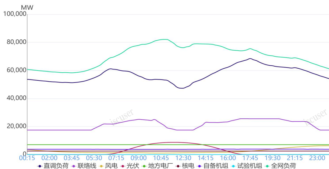
图 1 10月27日负荷及电源出力预测情况
