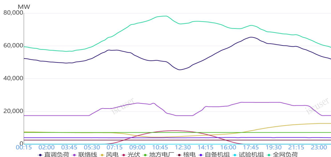
图 1 10月29日负荷及电源出力预测情况
