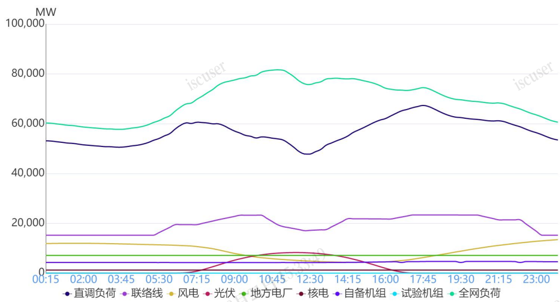
图 1 11月1日负荷及电源出力预测情况
