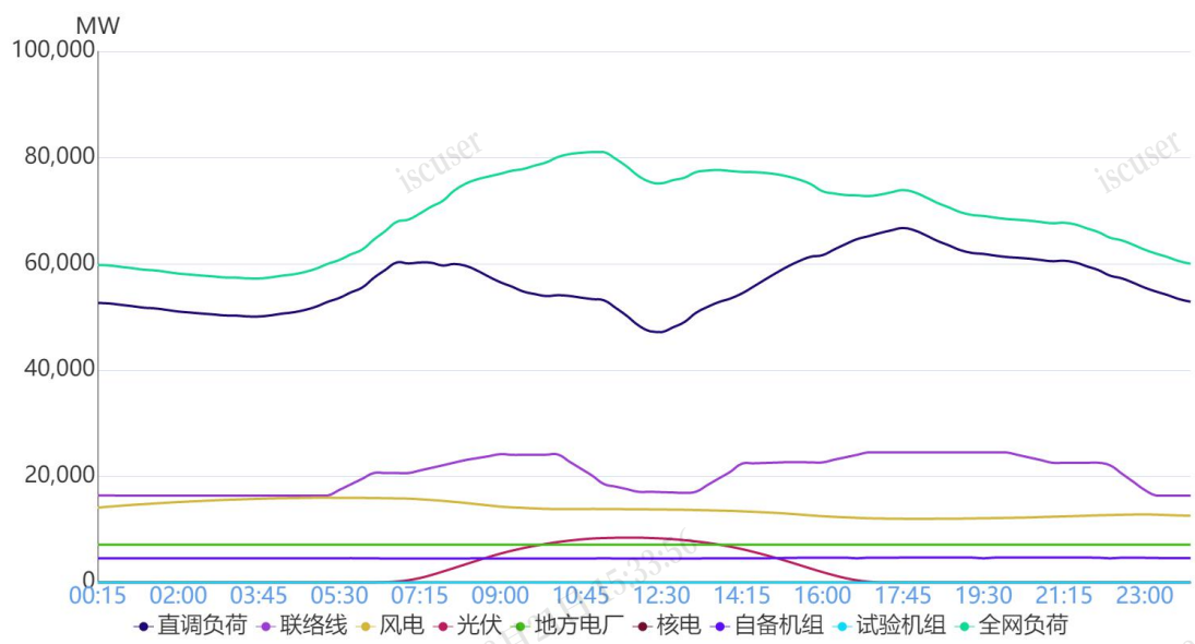
图 1 11月2日负荷及电源出力预测情况
