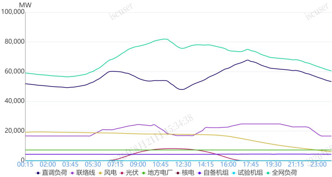
图 1 11月6日负荷及电源出力预测情况
