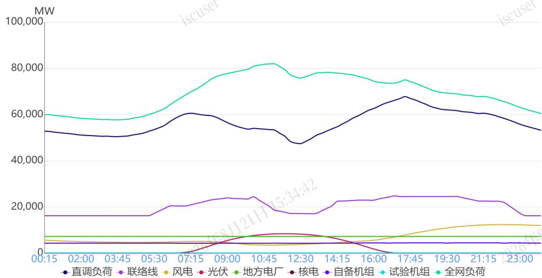
图1 11月7日负荷及电源出力预测情况
