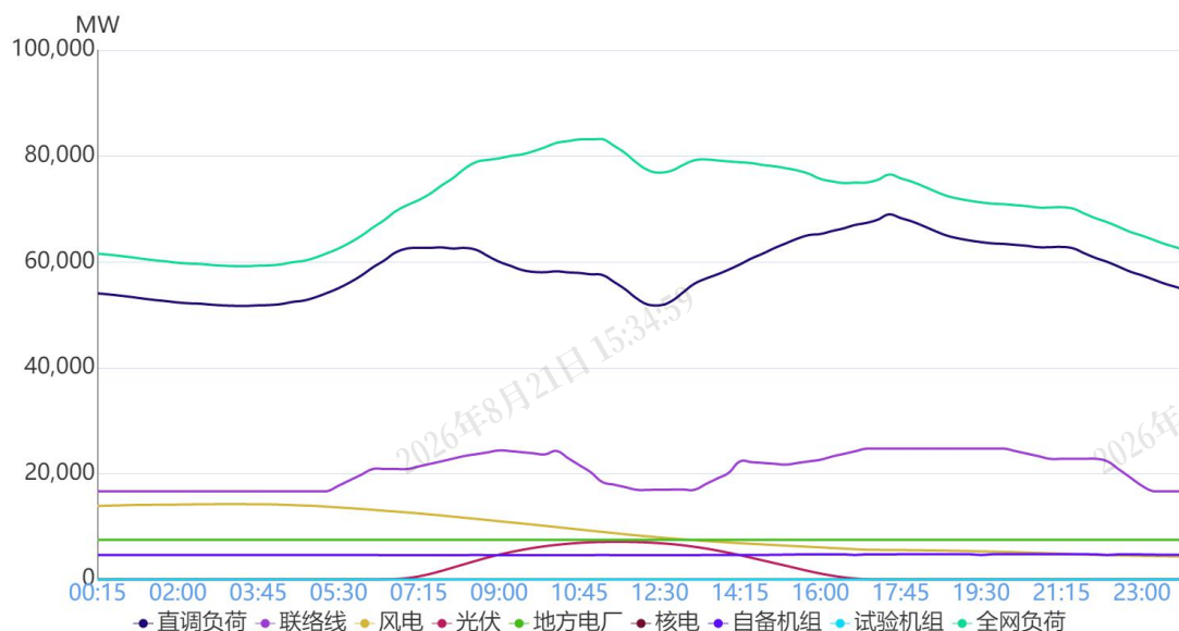
图1 11月10日负荷及电源出力预测情况
