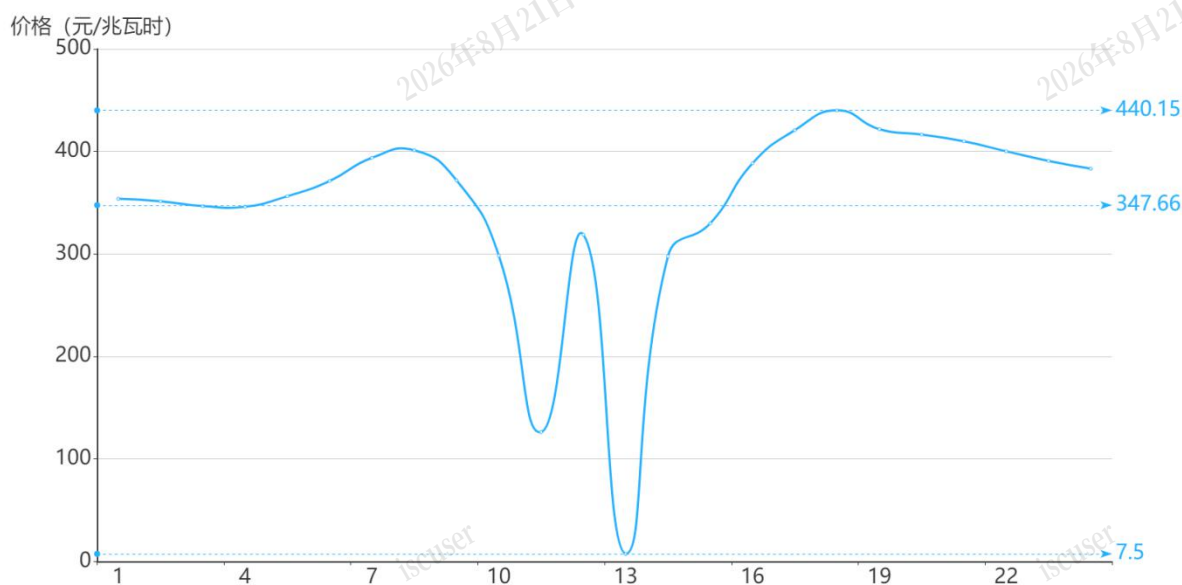
图3 11月13日实时市场用电侧价格
