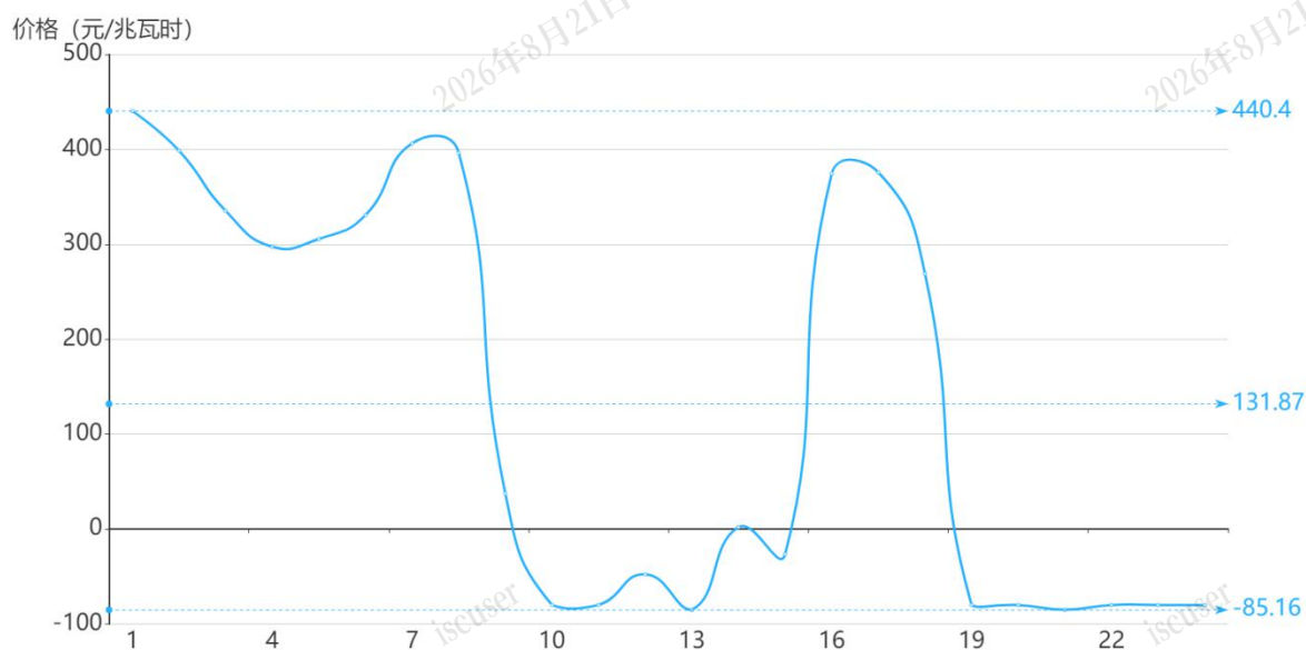
图3 11月20日实时市场用电侧价格
