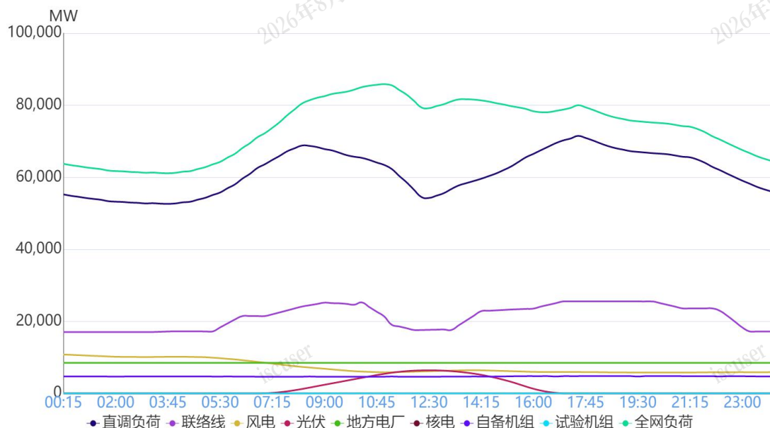
图 1 11月22日负荷及电源出力预测情况
