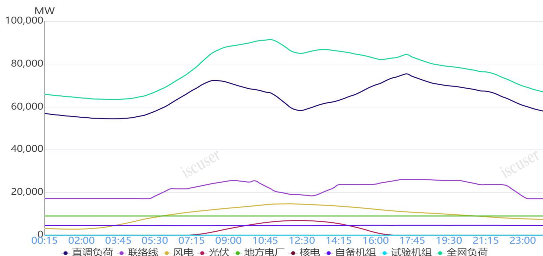
图 1 11月29日负荷及电源出力预测情况
