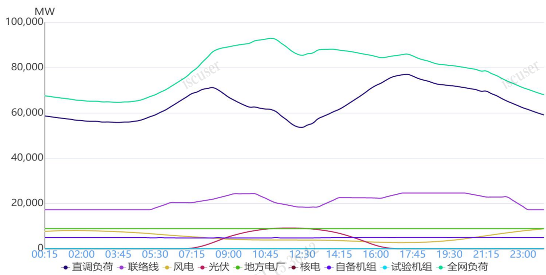
图 1 12月1日负荷及电源出力预测情况
