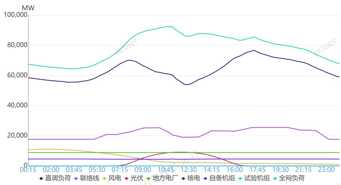
图 1 12月2日负荷及电源出力预测情况
