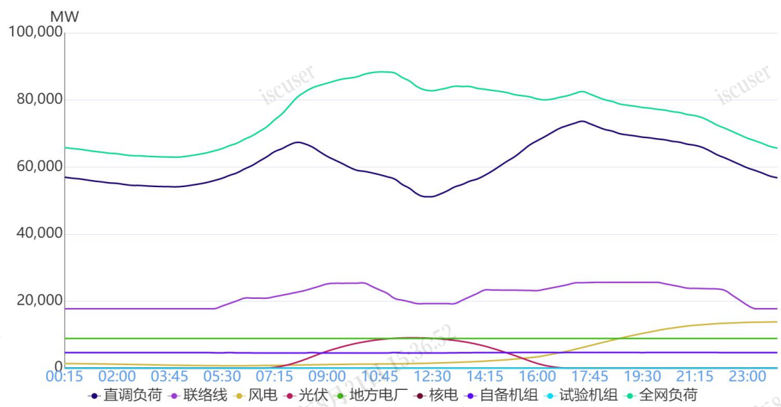
图 1 12月3日负荷及电源出力预测情况
