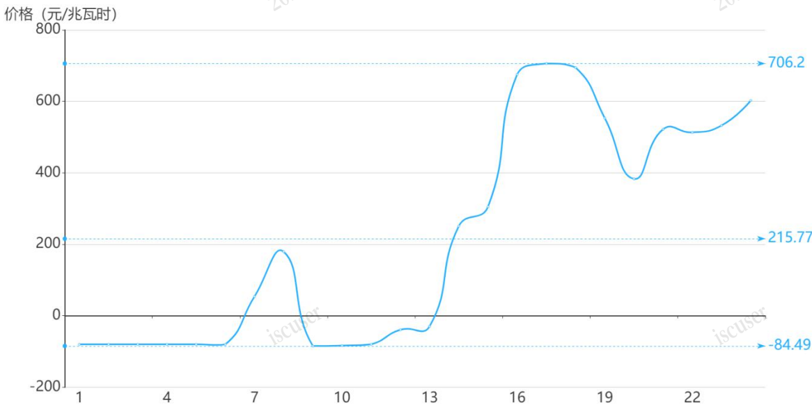
图 3 12 月 4 日实时市场用电侧价格
