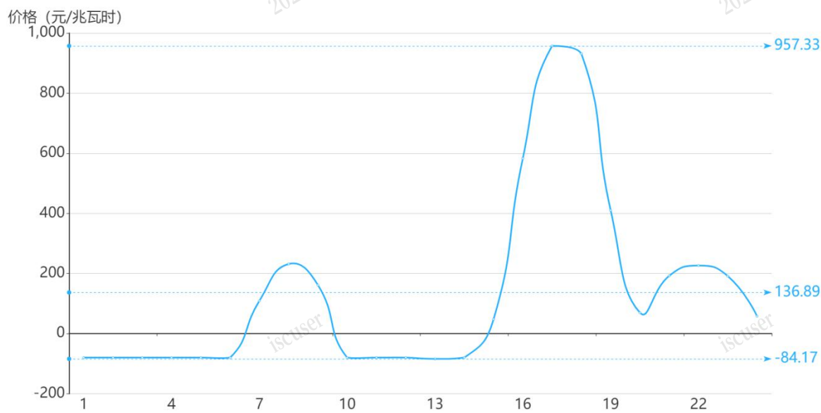
图 3 12 月 6 日实时市场用电侧价格
