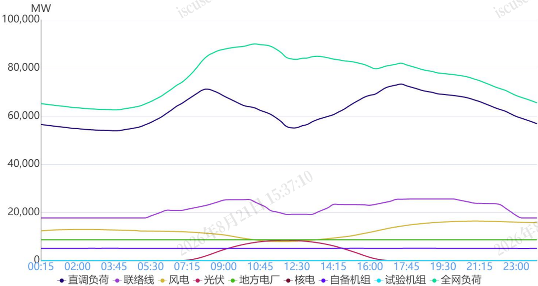
图 1 12月7日负荷及电源出力预测情况
