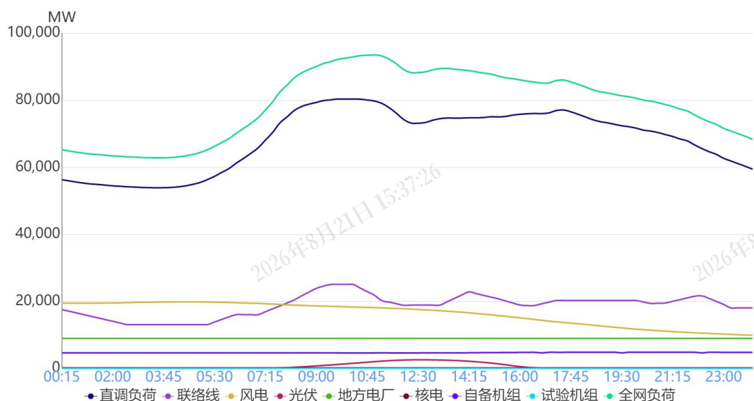
图 1 12月11日负荷及电源出力预测情况
