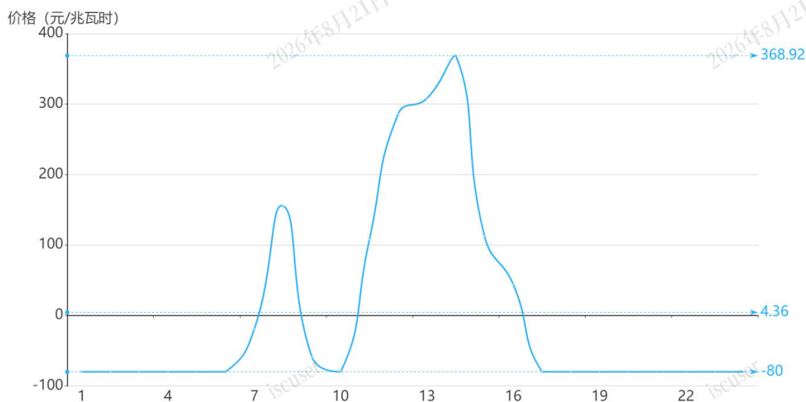
图3 12月10日实时市场用电侧价格
