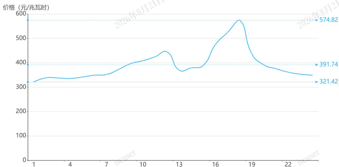
图3 12月12日实时市场用电侧价格
