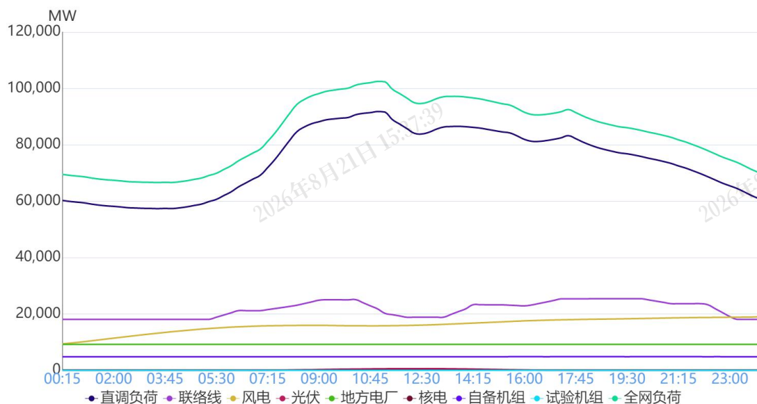
图1 12月14日负荷及电源出力预测情况
