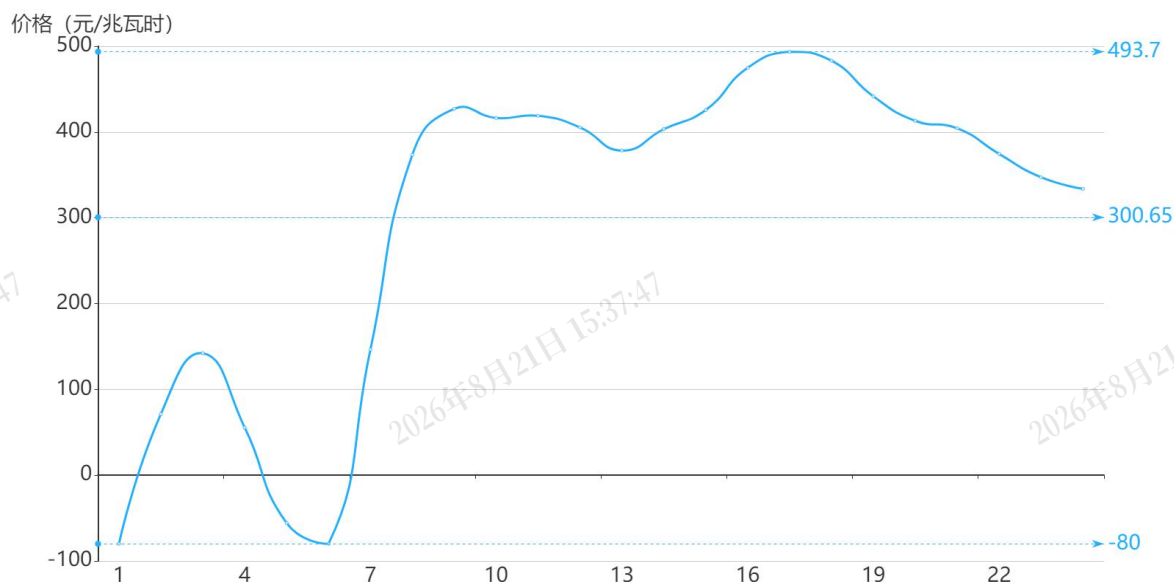
图 2 12 月 16 日日前市场用电侧价格
