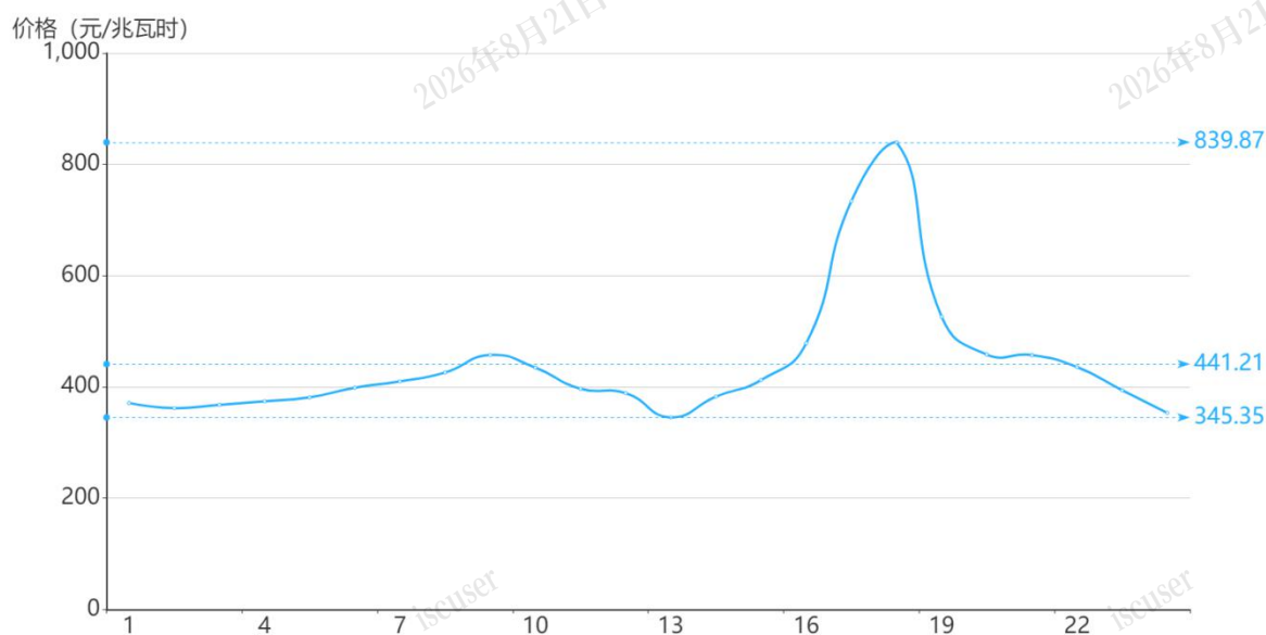
图3 12月23日实时市场用电侧价格
