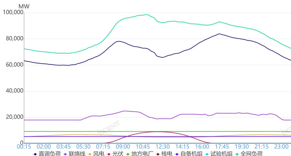
图 1 12月24日负荷及电源出力预测情况
