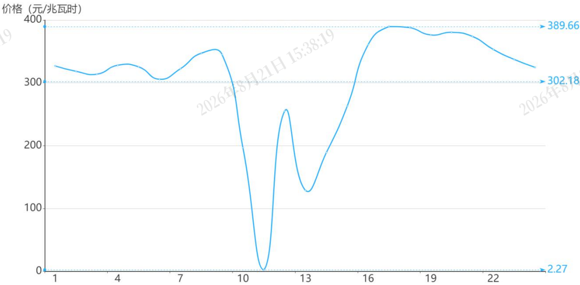
图 2 12 月 24 日日前市场用电侧价格
