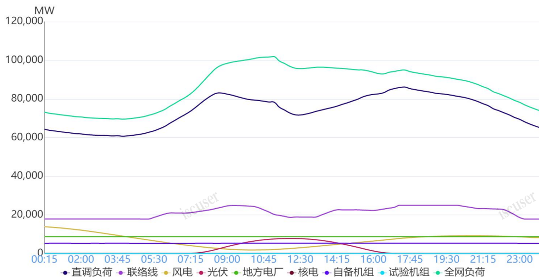
图 1 12月26日负荷及电源出力预测情况
