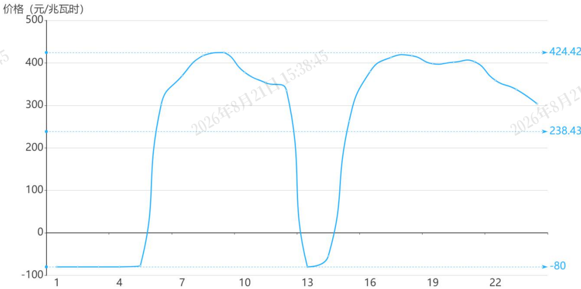
图 2 12 月 26 日日前市场用电侧价格
