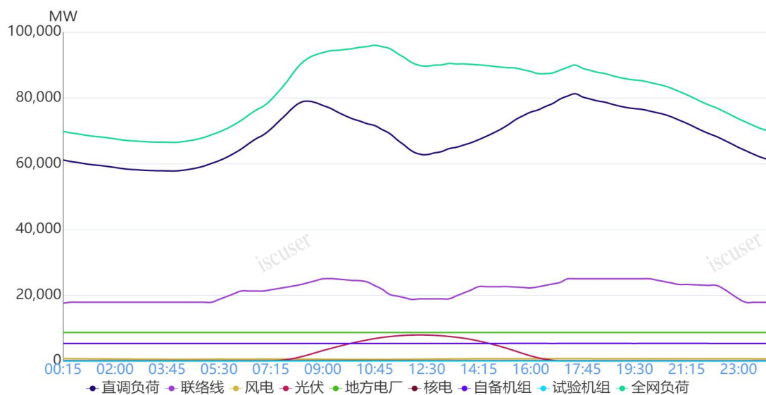
图 1 12月28日负荷及电源出力预测情况
