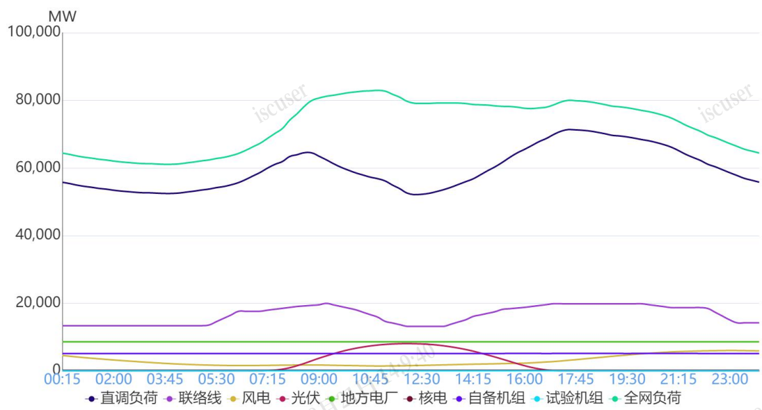
图 2 1月1日负荷及电源出力预测情况
