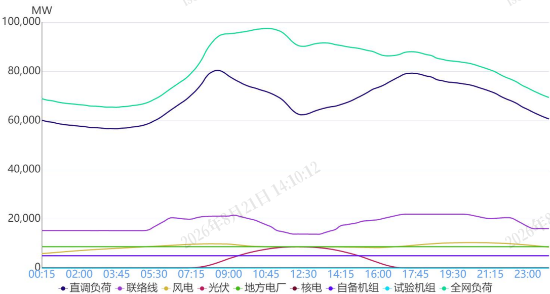
图 1 1月8日负荷及电源出力预测情况
