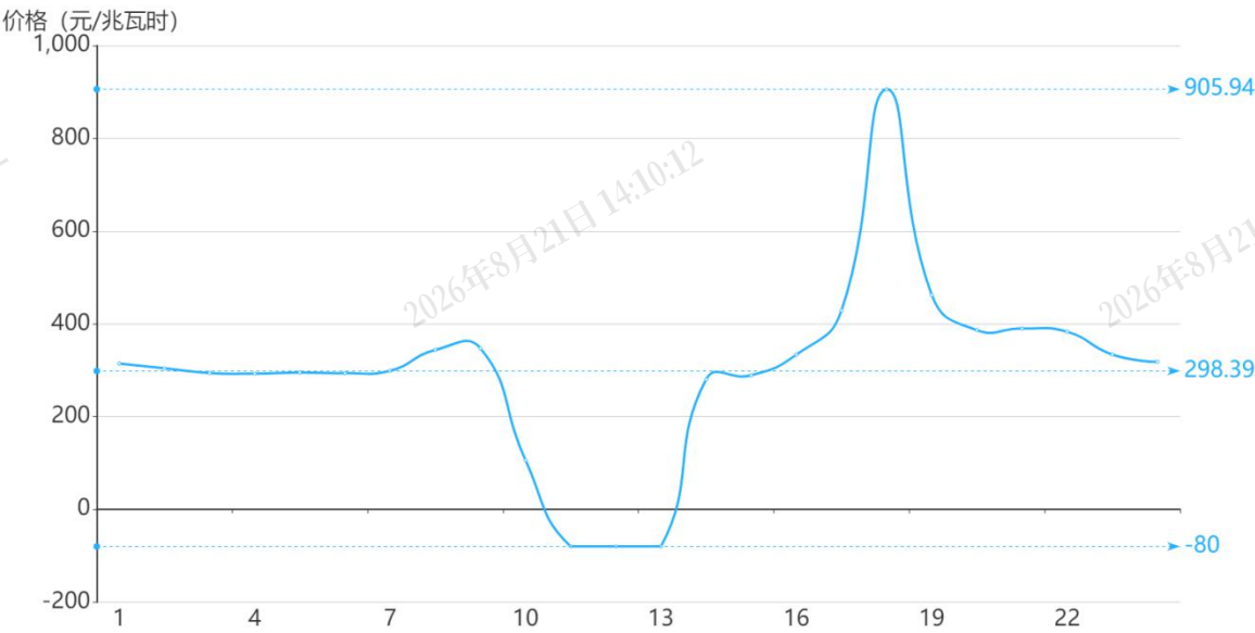
图 3 1 月 7 日实时市场用电侧价格
