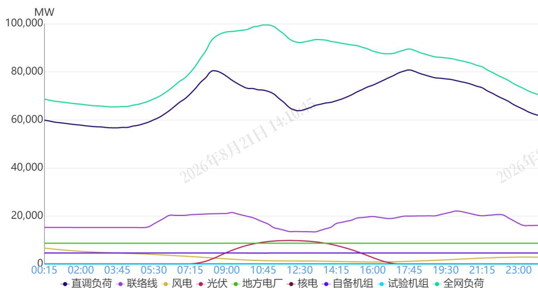
图1 1月15日负荷及电源出力预测情况
