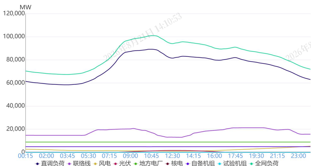
图1 1月17日负荷及电源出力预测情况
