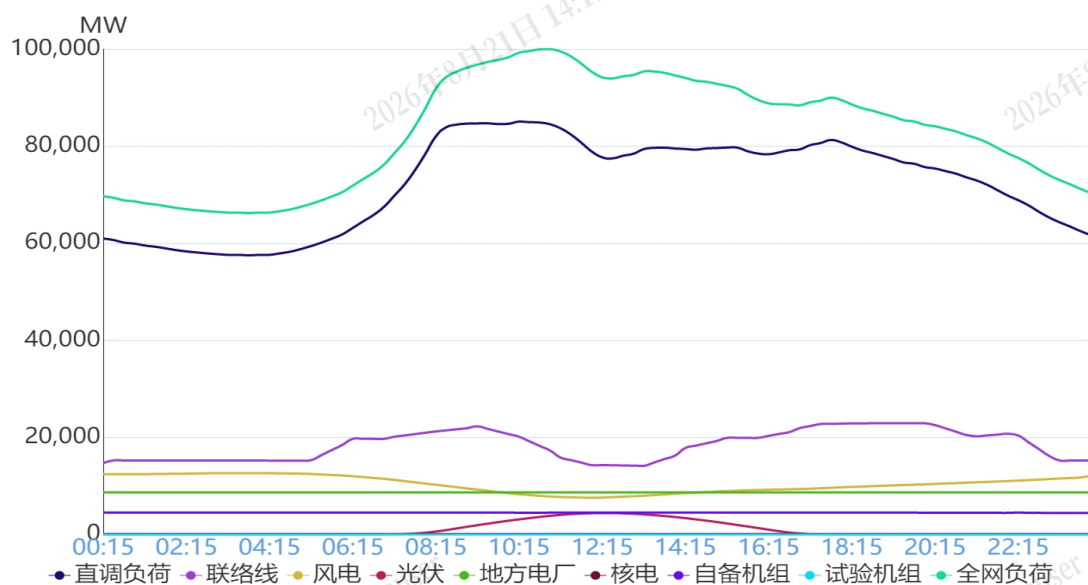
图1 1月20日负荷及电源出力预测情况
