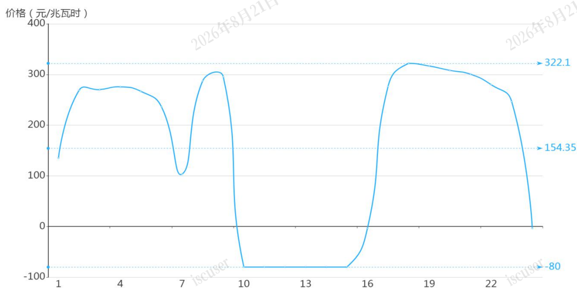
图3 1月21日实时市场用电侧价格
