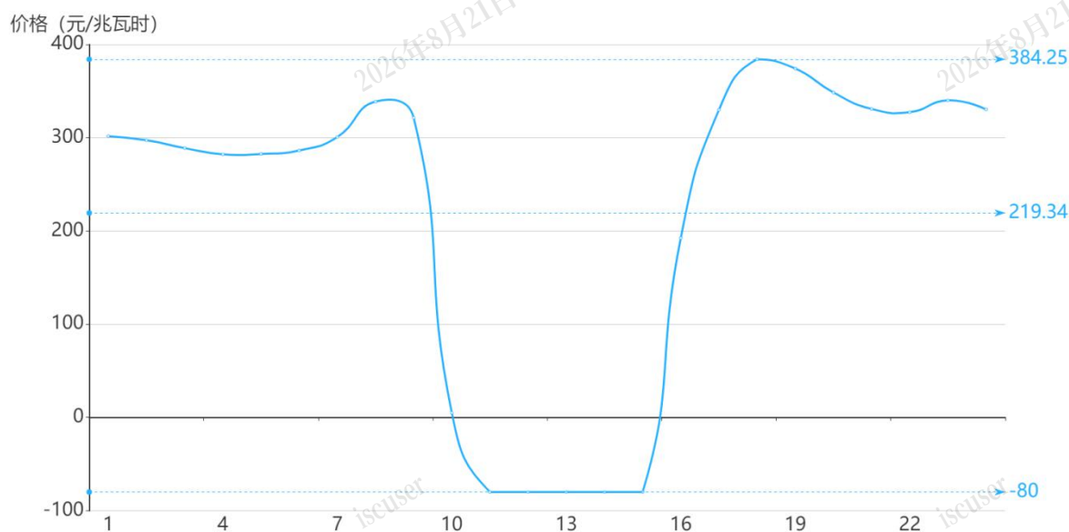
图3 1月26日实时市场用电侧价格
