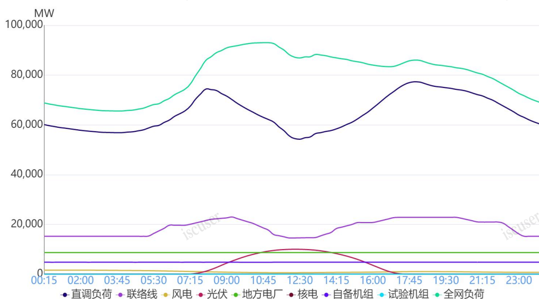
图 1 1月27日负荷及电源出力预测情况
