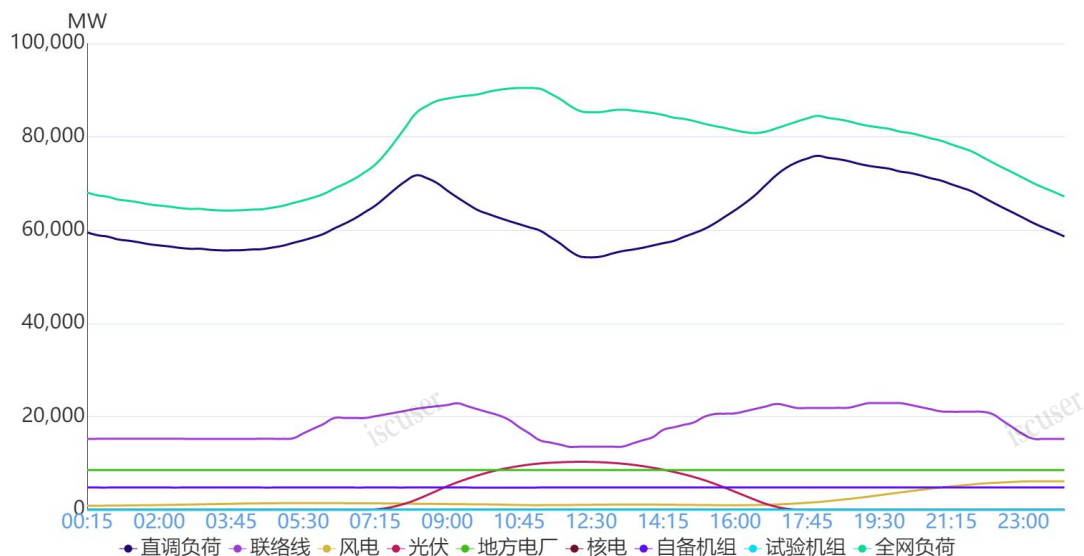
图 1 1月28日负荷及电源出力预测情况
