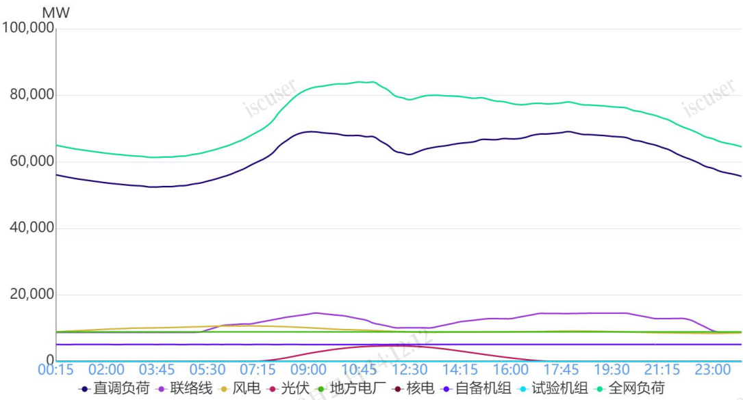
图 1 2月4日负荷及电源出力预测情况
