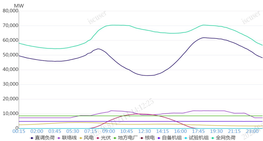
图 1 2月7日负荷及电源出力预测情况
