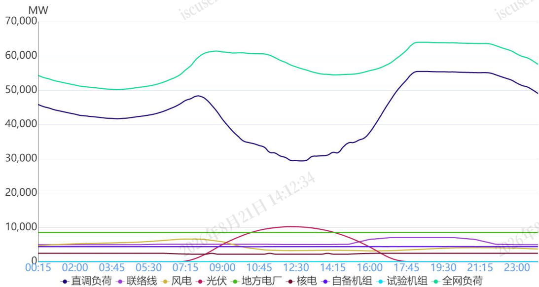
图 1 2月9日负荷及电源出力预测情况
