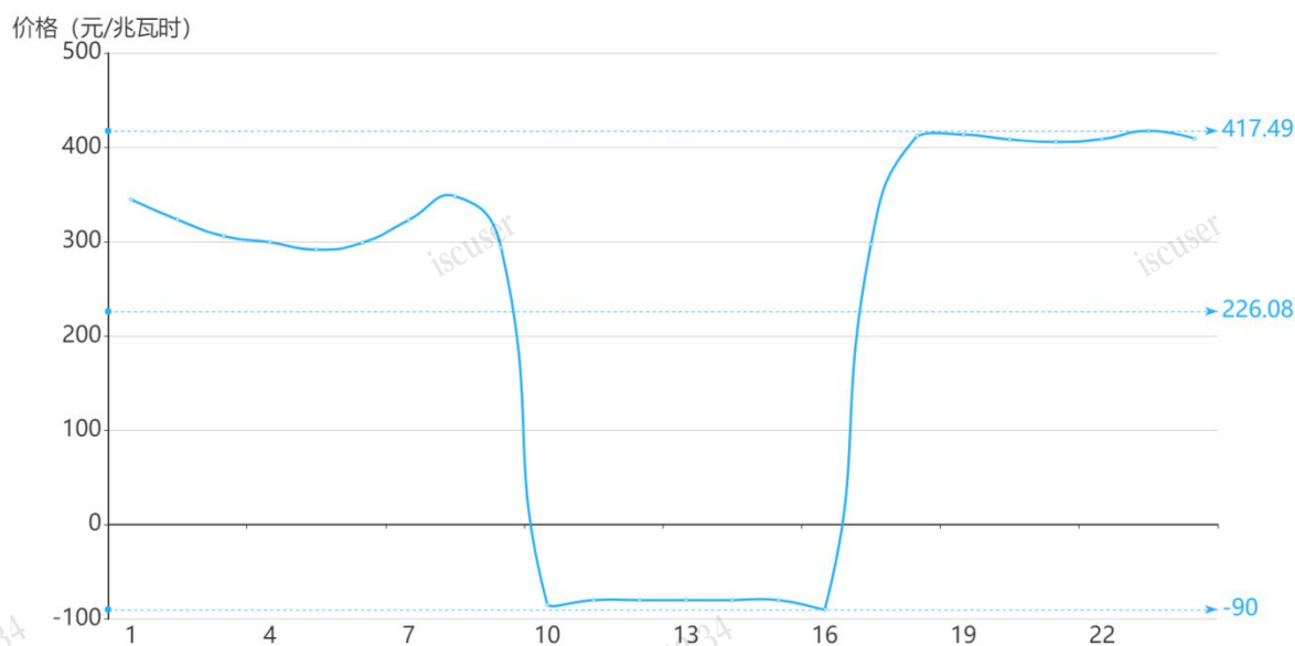
图2 2月9日日前市场用电侧价格
