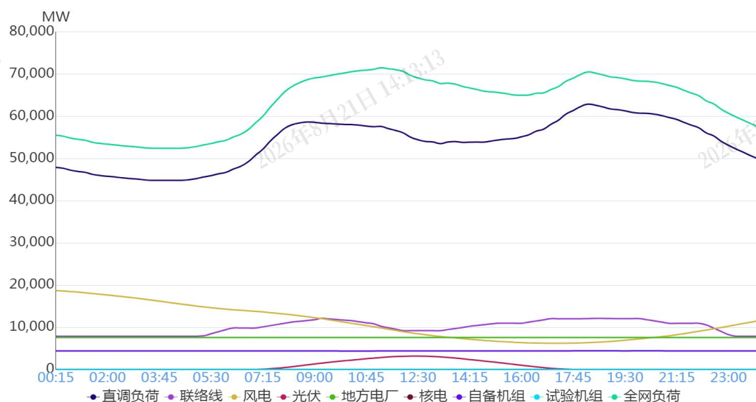
图 1 2月18日负荷及电源出力预测情况
