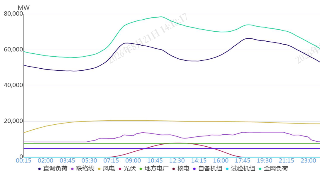
图 1 2月19日负荷及电源出力预测情况
