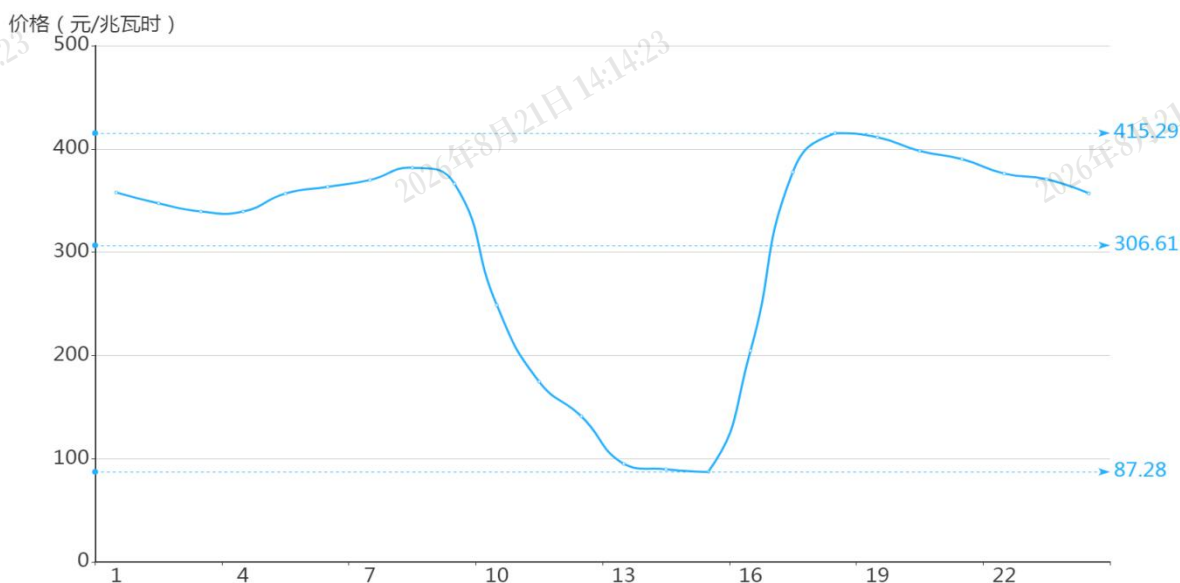
图 2 2 月 27 日日前市场用电侧价格
