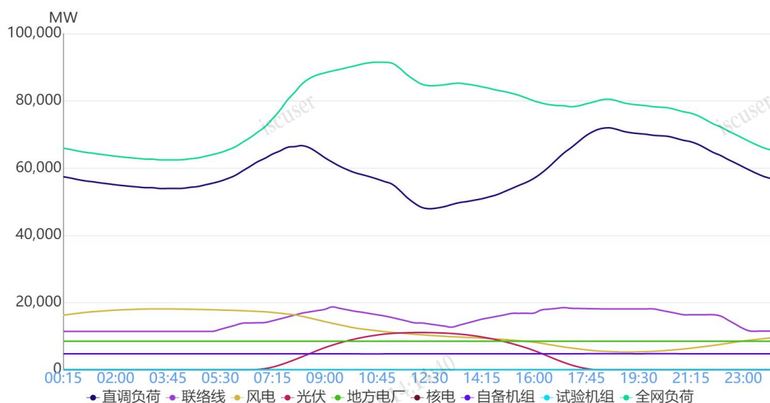
图1 3月2日负荷及电源出力预测情况
