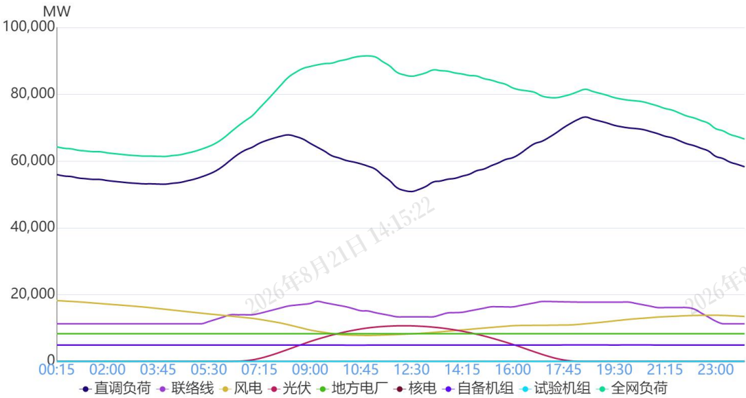
图 1 3月11日负荷及电源出力预测情况
