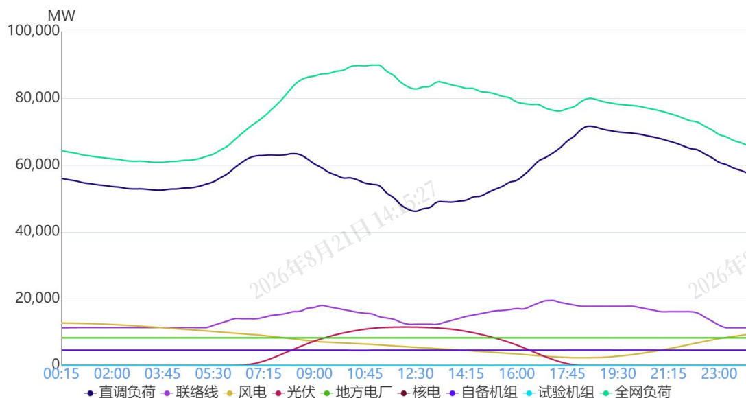
图1 3月12日负荷及电源出力预测情况
