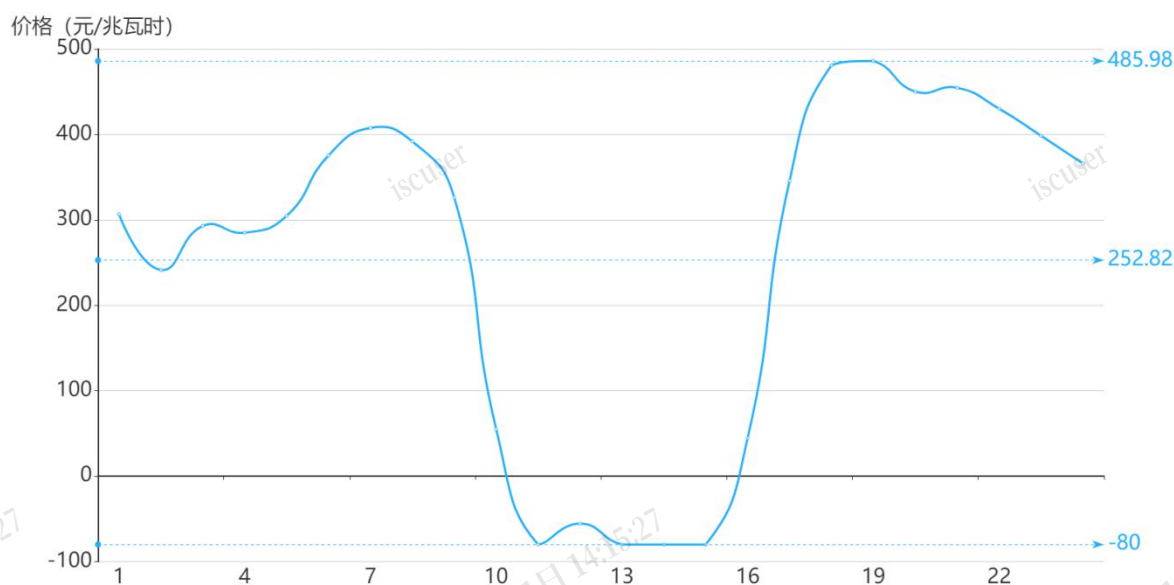
图 2 3 月 12 日日前市场用电侧价格
